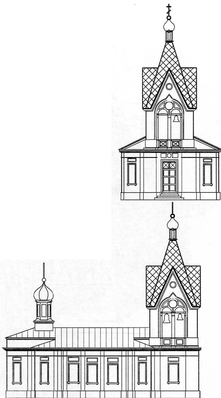
II. 4 Elewacja główna i boczna cerkwi prawosławnej w Surażu-wg projektu zatwierzonego 11 listopada 1864 roku-zob. Państwowe Archiwum Historyczne Białorusi w Grodnie F. 97, op. 1 nr. 32 k. 55.
