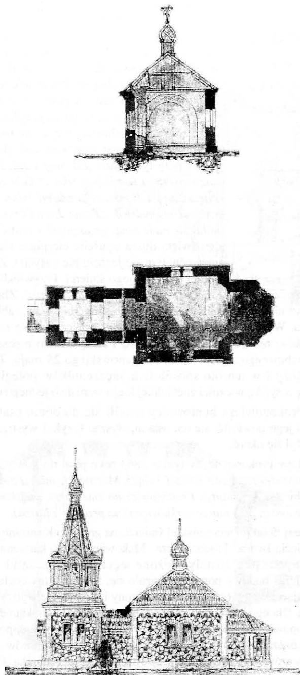
Il. 5 Drukowany, typowy projekt cerkwi prawosławnej dla 200 osób, proponowany do zbudowania w Surazu por. Państwowe Archiwum Historyczne Białorusi w Grodnie, F. 97, op. 1 nr 32, k. 89-90
