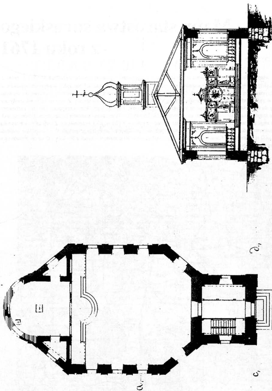
Plan i przekrój projektowanej cerkwi w Surażu-1864 r. Państwowe Muzeum Historyczne w Grodnie F. 97, op. I, nr 32 k. 56
